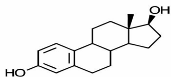
Estradiol
