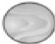
Venus
