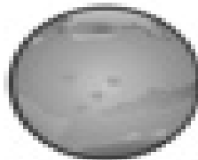
Mars
