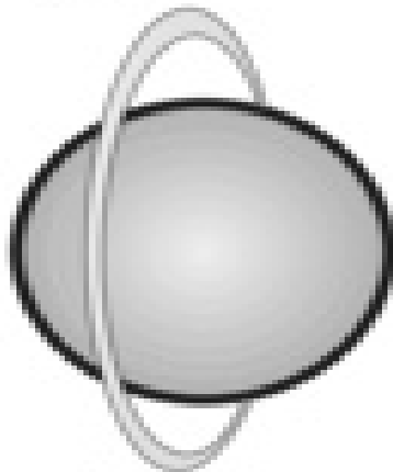
Uranus
