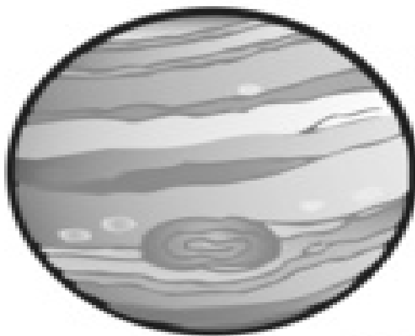
Jupiter
