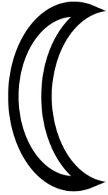
Moon
