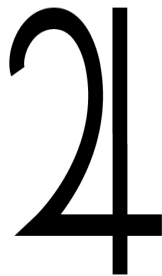
Jupiter
