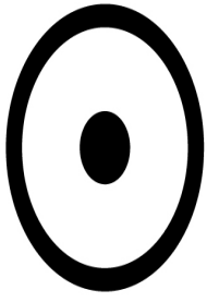
Sun
