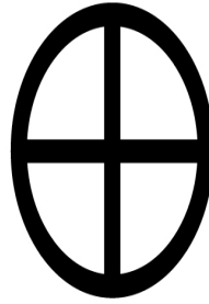
Earth
