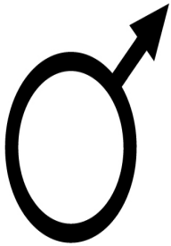
Mars
