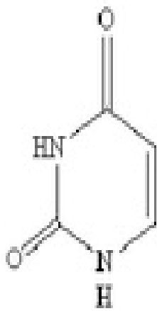
Uracil
