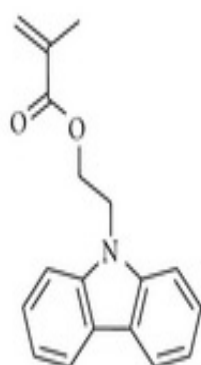
CzEMA
