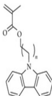
CzAMA
