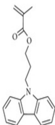
CzPMA
