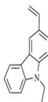
E3VC
