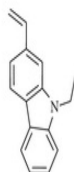
E2VC
