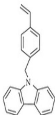
VBCz
