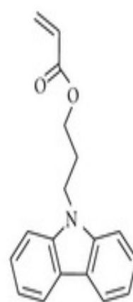
CzPA
