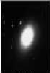
M84 Elliptical, E1
