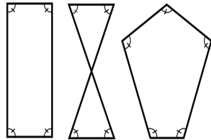
Equiangular
