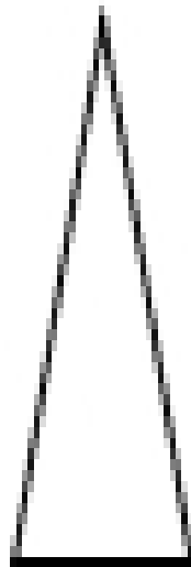
Isosceles
