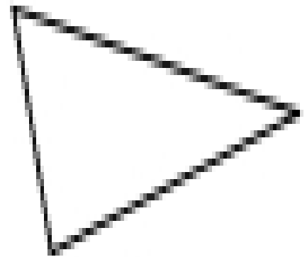
Scalene
