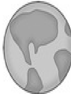
Earth
