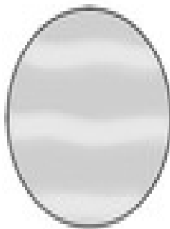
Venus
