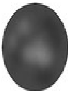
Mars
