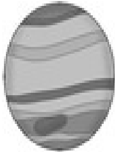
Jupiter
