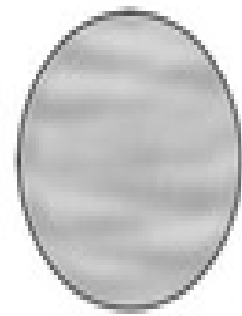
Uranus
