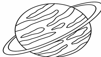
Uranus
