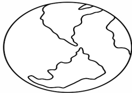
Earth
