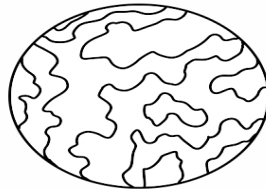
Mars
