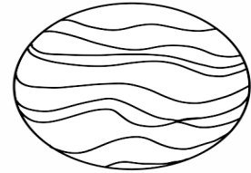
Venus
