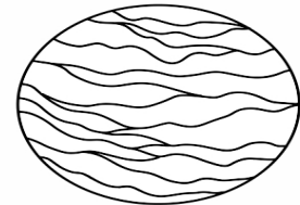
Jupiter
