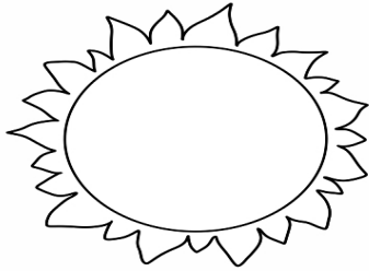
Sun
