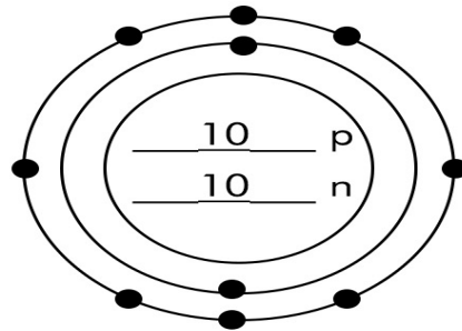
Neon-20
