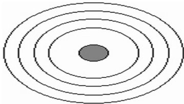
Calcium
