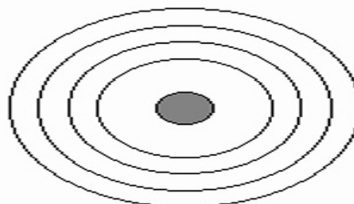
Helium
