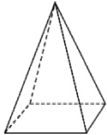
Pyramid
