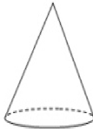
Cone
