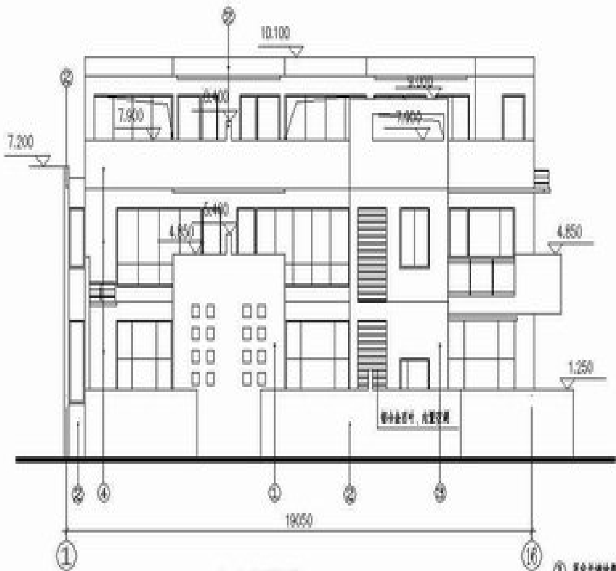
南立面图
