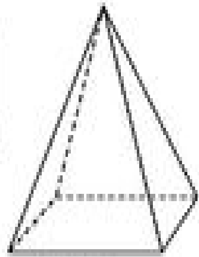
Pyramid
