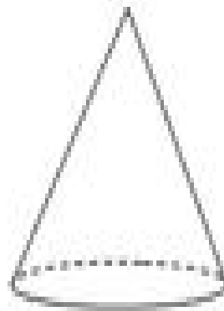
Cone
