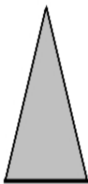
Acute isosceles
