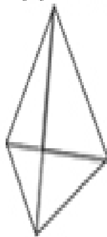
pyramid
