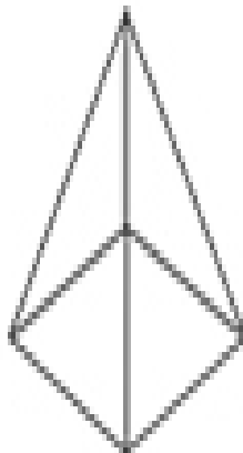
pyramid
