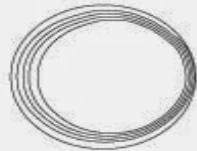
Mars
