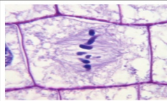
METAPHASE
