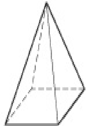
Pyramid
