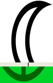
Earth
