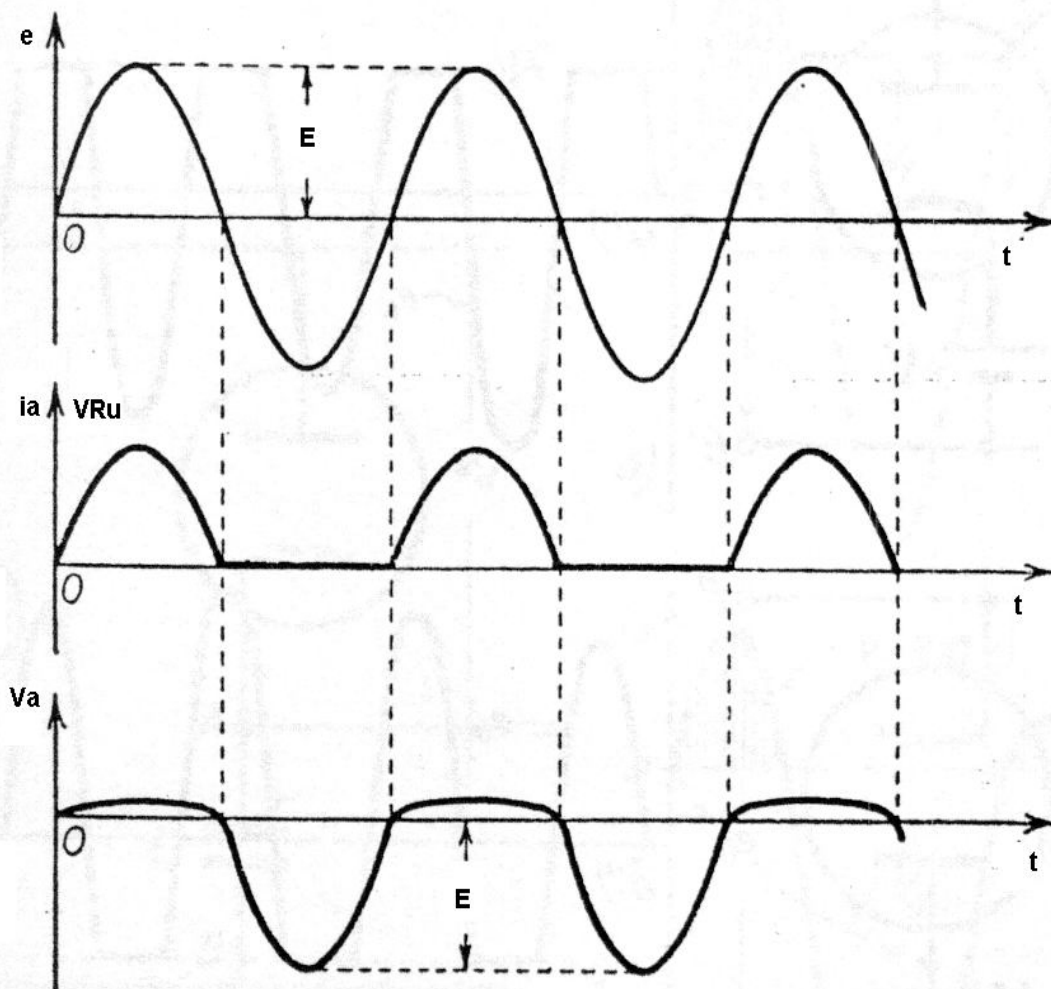
— Diagrammi significativi delle tensioni e correnti nel raddrizzatore a diodo.
