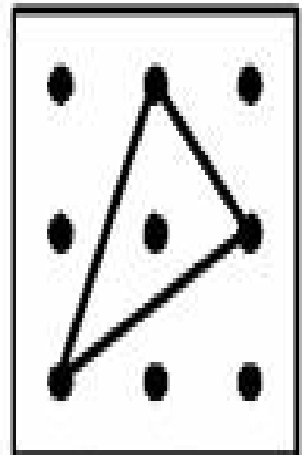
isosceles
