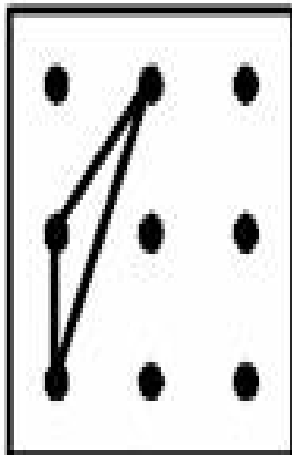
scalene
