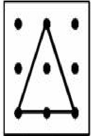
isosceles
