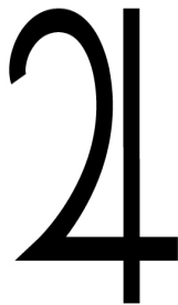
Jupiter
