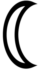
Moon
