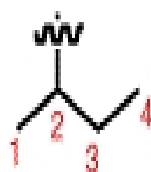
2-butyl
