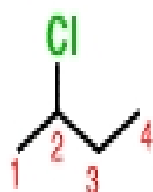
2-butyl chloride
