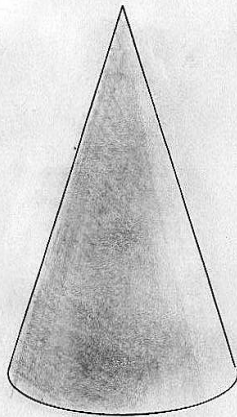
Cone
