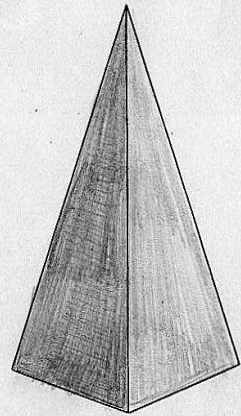
Pyramid
