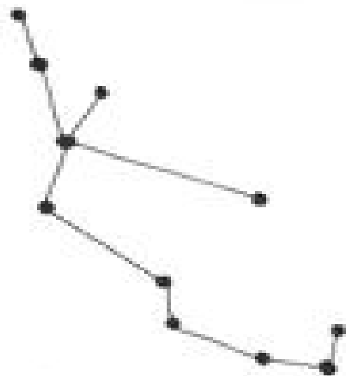
Perseus
