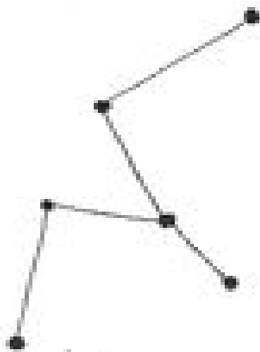
Aquila
