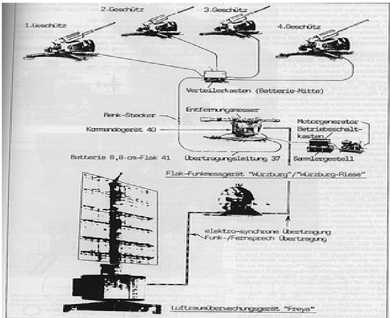
Funkmessgesteuertes Flaksystem mit einer Batterie 8,8-cm-Flak 41
