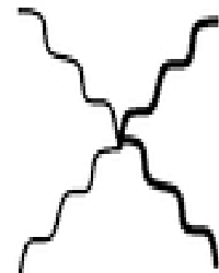
Dumbbell (pom-pom)
