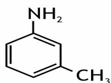
3-aminotoluene
