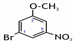
1-bromo-3-methoxy-5-nitrobenzene
