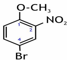
4-bromo-1-methoxy-2-nitrobenzene
