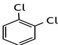
1,2-dichlorobenzene
