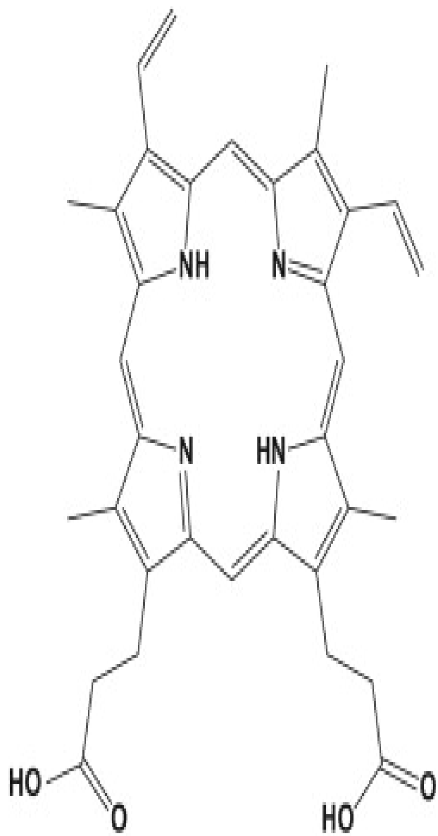
Protoporphyrin IX
