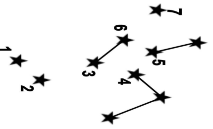
Hercules
